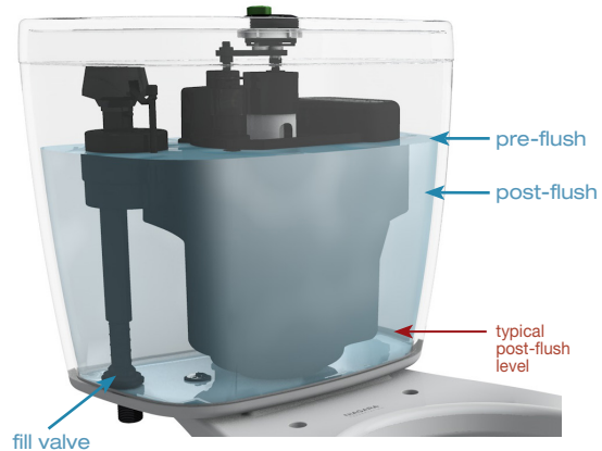
fill valve
